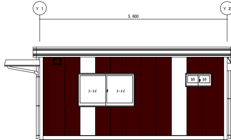
X 2 立面図 S=1/50
