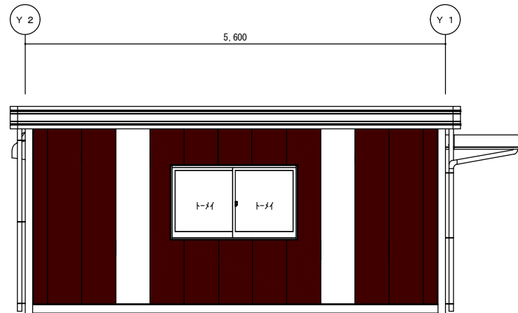
X 1 立面図 S=1/50
