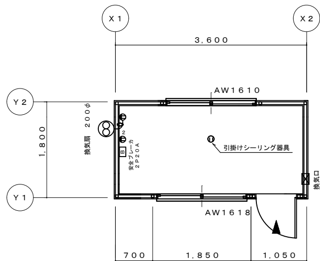
平面図 S=1/50
