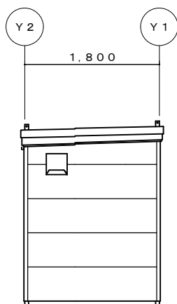
X1立面図 S=1/50
