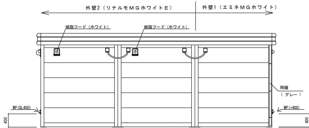
A 立面図
