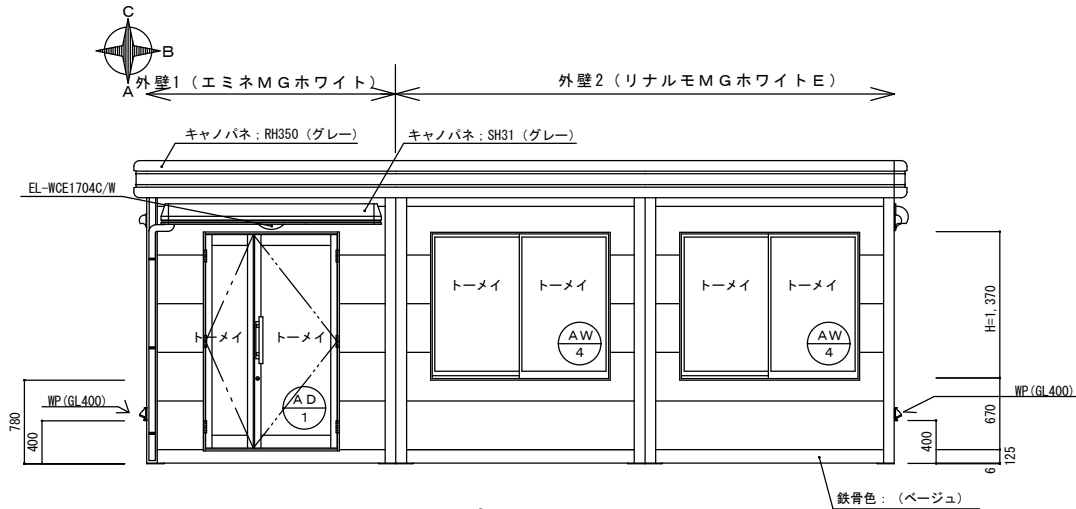
A 立面図
