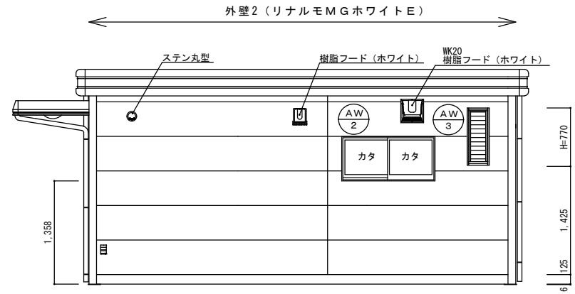
B 立面図
