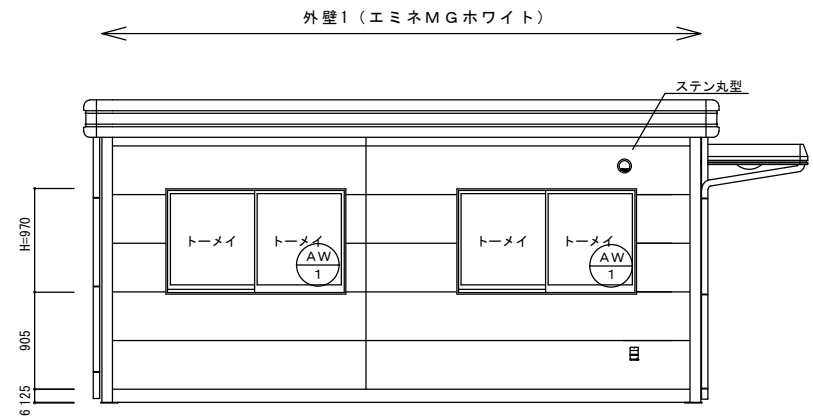
D 立面図
