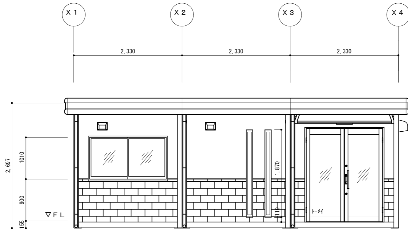
Y 1 立面図 S = 1 / 5 0
