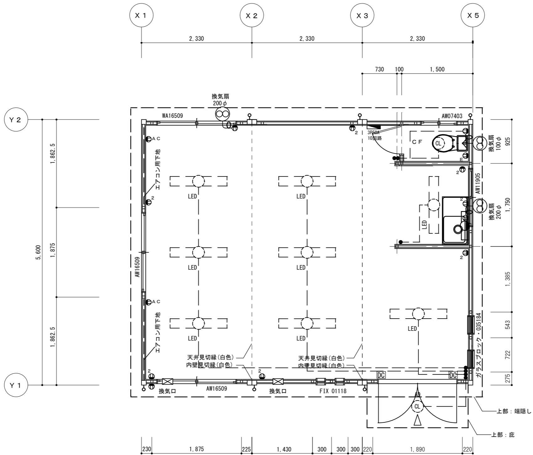
平面図 S = 1 / 50
