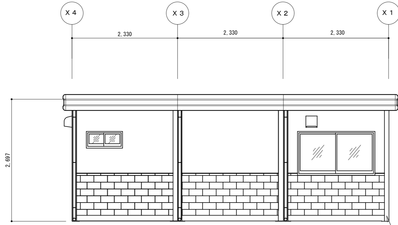
Y 2 立面図 S = 1 / 5 0
