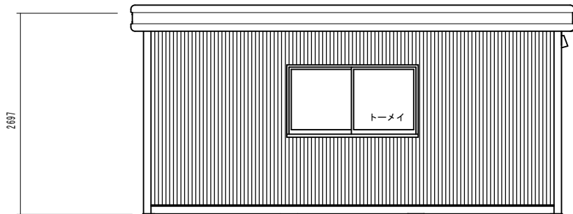
X2 - 立面図 S=1/50
