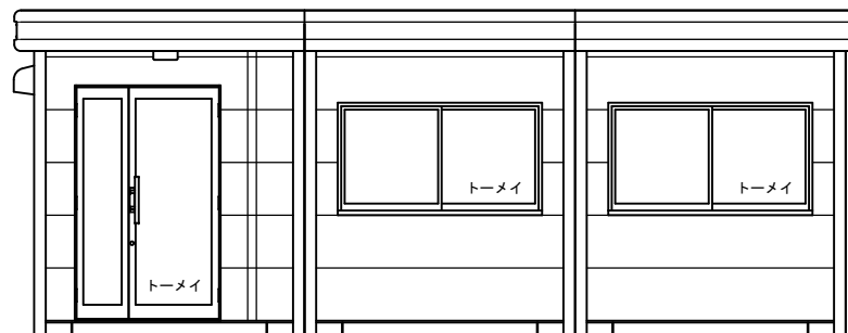
Y1 - 立面図 S=1/50
