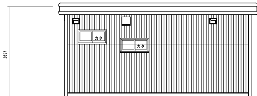
X1 - 立面図 S=1/50
