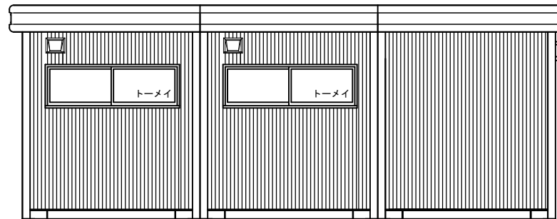
Y2 - 立面図 S=1/50
