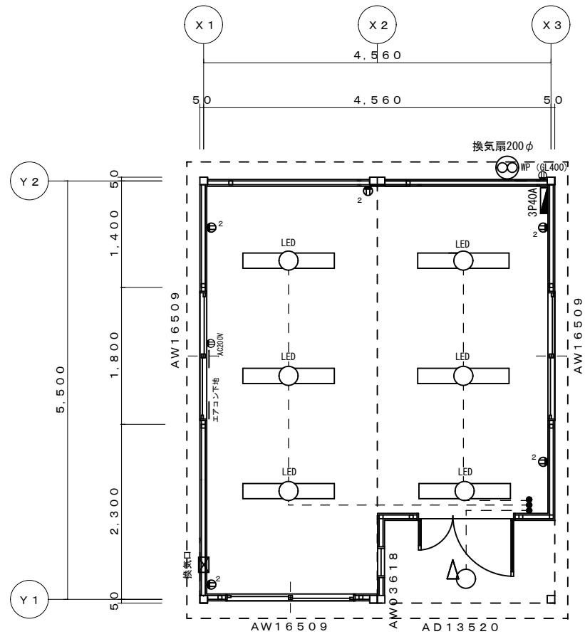
平面図 S = 1/50
