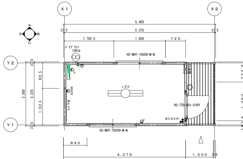
平面図 S = 1 / 50
