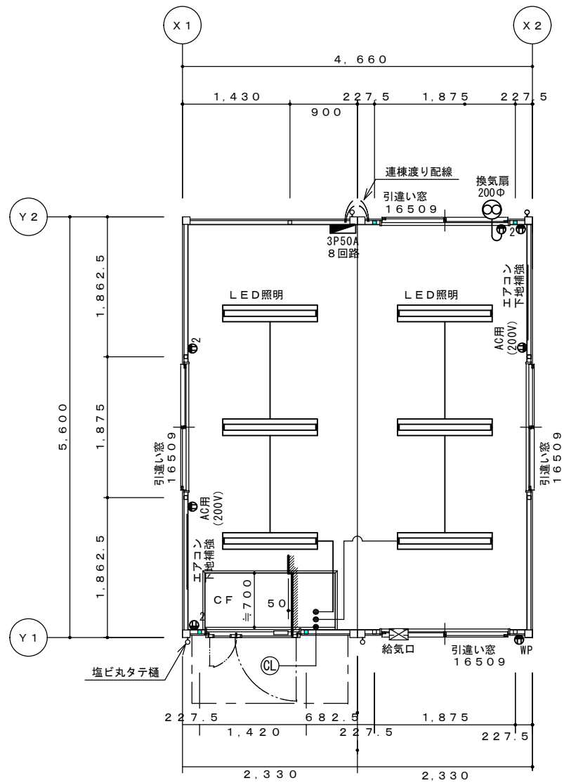
平面図 S = 1/50
