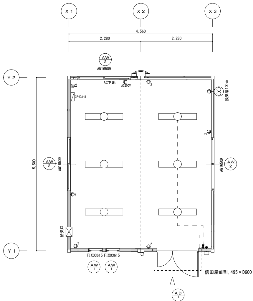
平面図 S = 1/50
