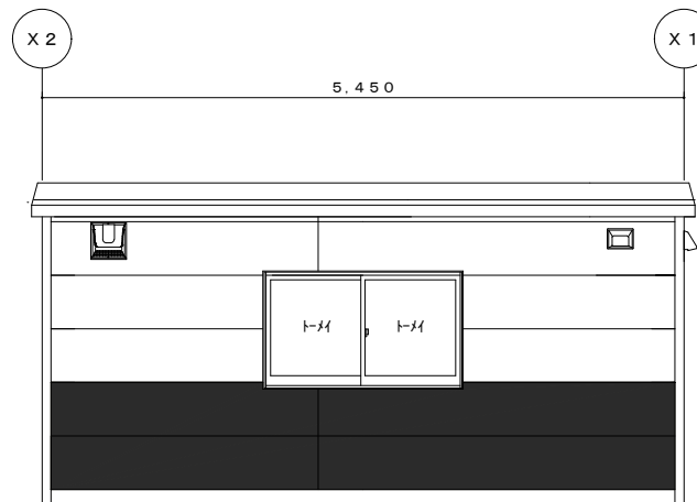
Y 2 立面図 S = 1 / 5 0
