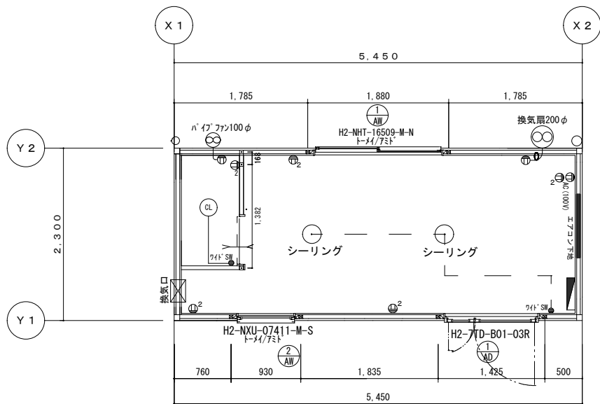
平面図 S = 1 / 5 0
