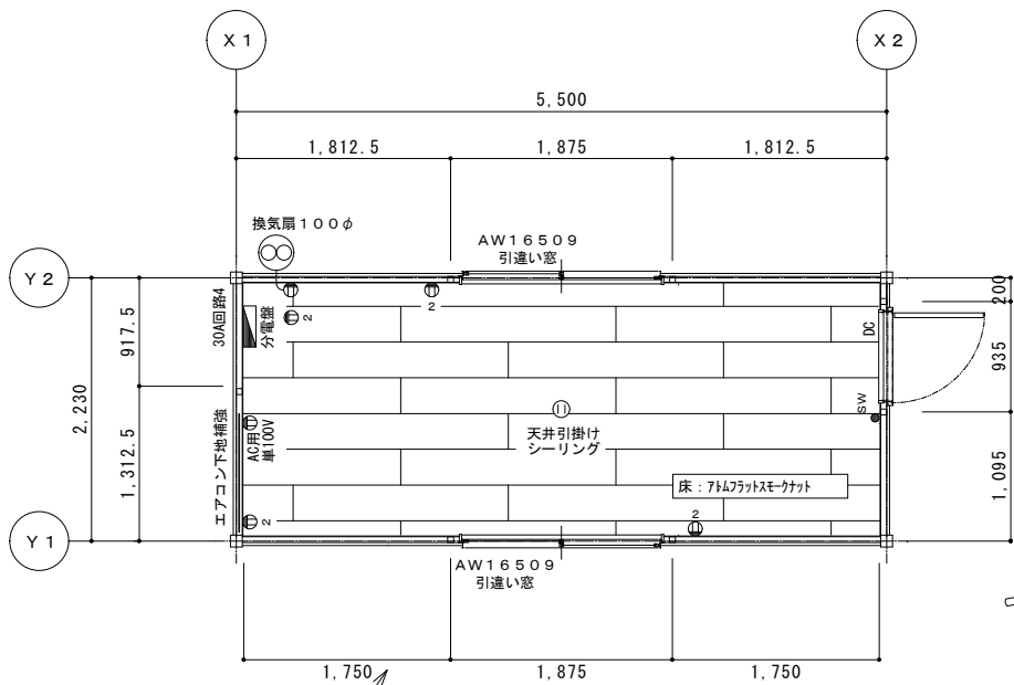
平面図 S=1/50
