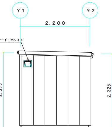
X2立面図 S=1/50
