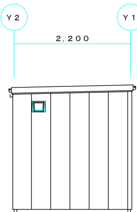
X1立面図 S=1/50
