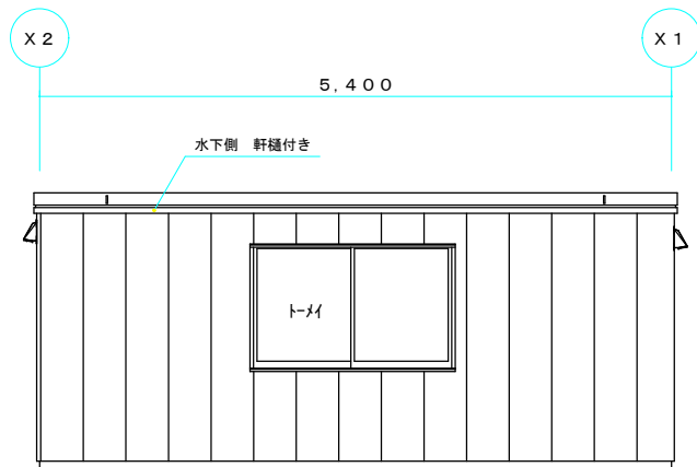
Y2立面図 S=1/50
