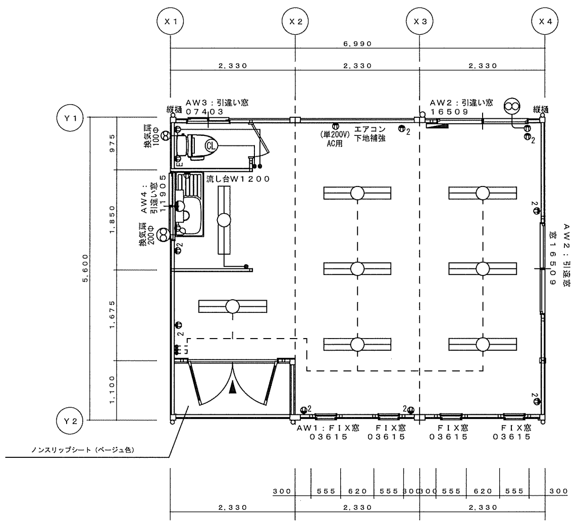
平面図 S = 1/50
