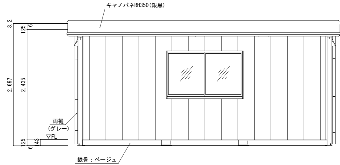
B側立面図 S = 1/50
