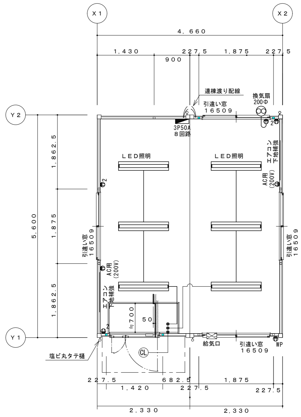
平面図 S = 1/50
