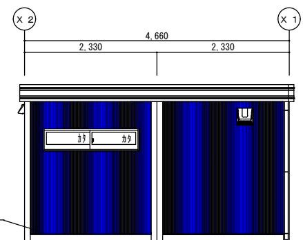
Y 2 立面図 S=1/50
