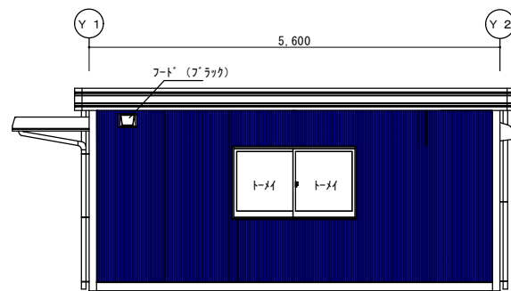
X 2 立面図 S=1/50
