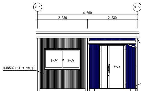
Y 1 立面図 S=1/50
