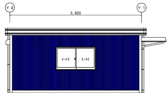
X 1 立面図 S=1/50
