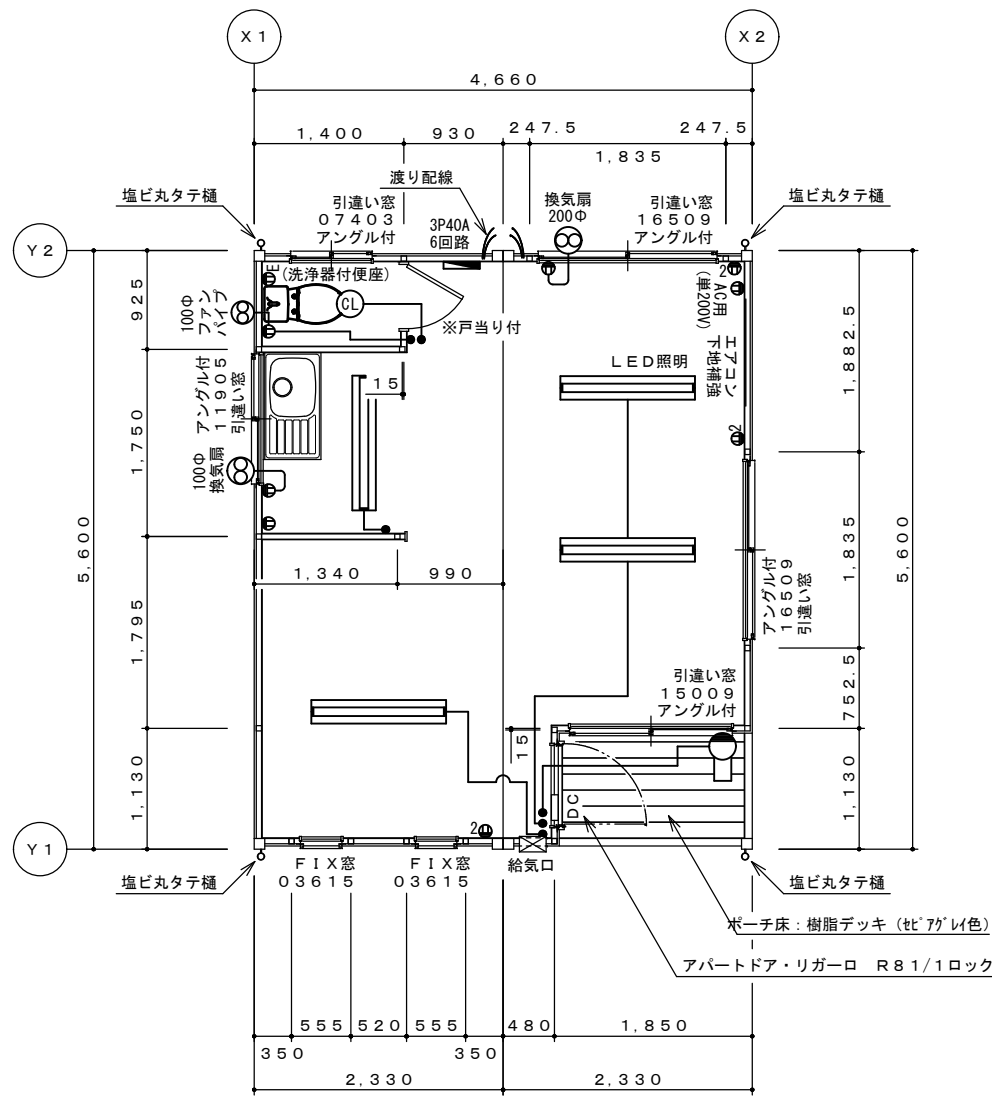
平面図 S=1/50
