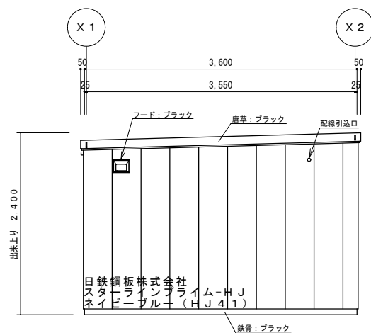
Y 1—立面图 S=1/50
