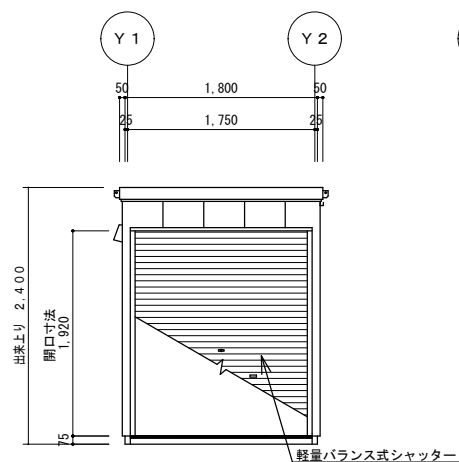
X 2-立面图 S=1/50
