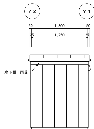
X 1—立面图 S=1/50
