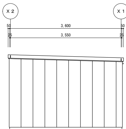
Y 2-立面图 S=1/50
