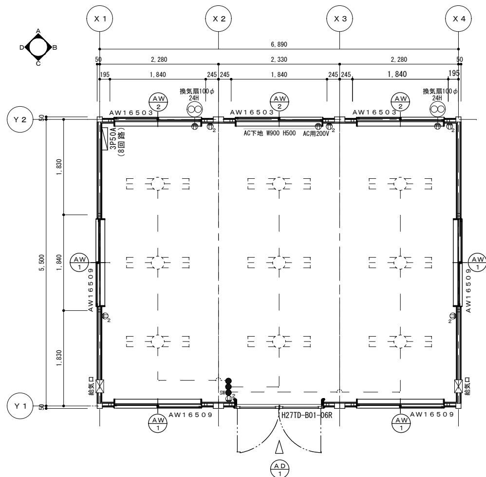
平面図 S = 1 / 5 0
