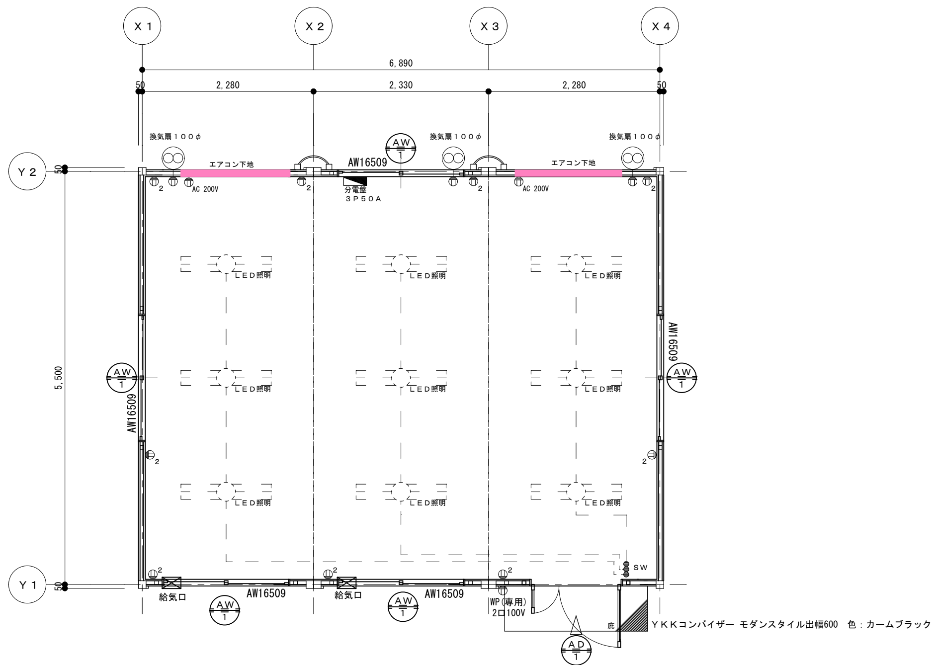
平面図 S=1/50
