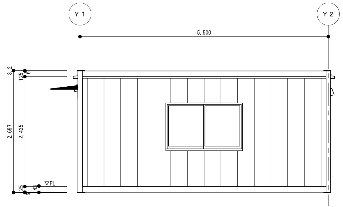
B側立面図 S = 1 / 5 0
