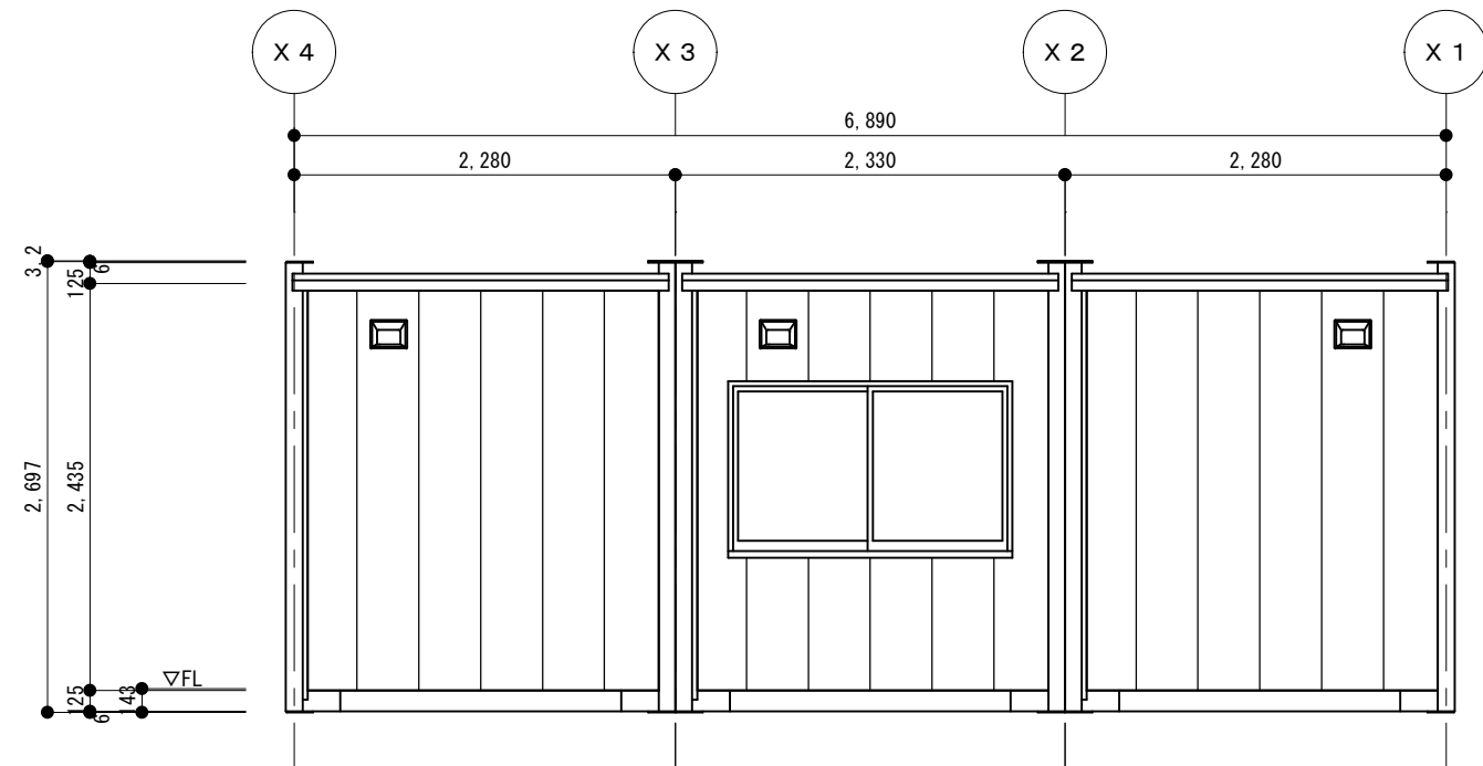
A側立面図 S = 1 / 5 0
