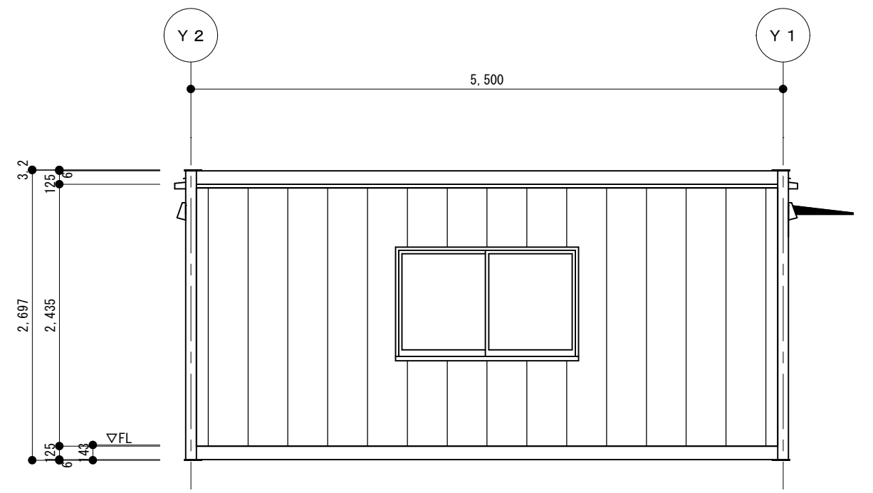
D側立面図 S = 1 / 5 0
