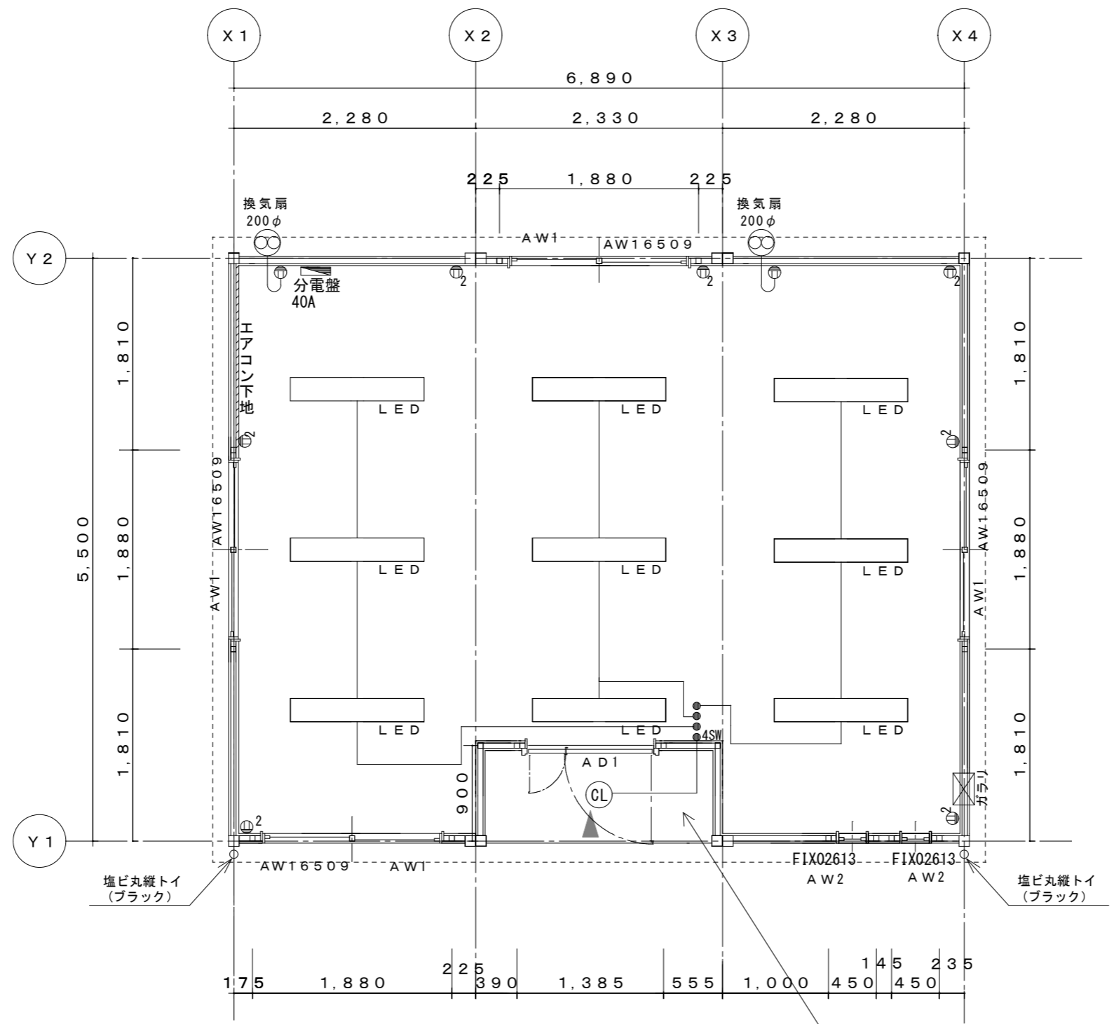
平面図 S = 1/50
