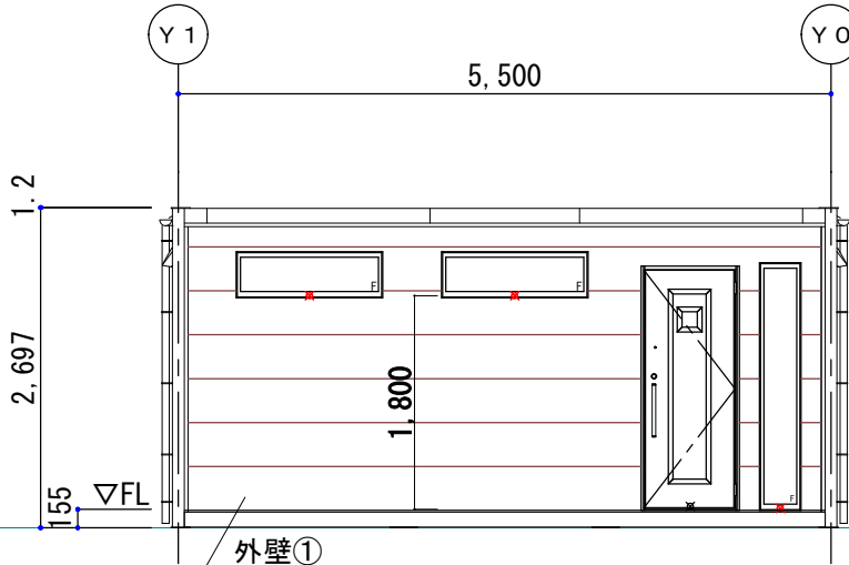
X0通り 1/100
