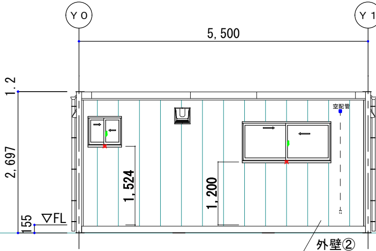
X3通り 1/100
