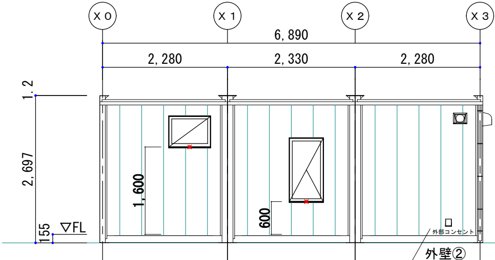
Y0通り 1/100
