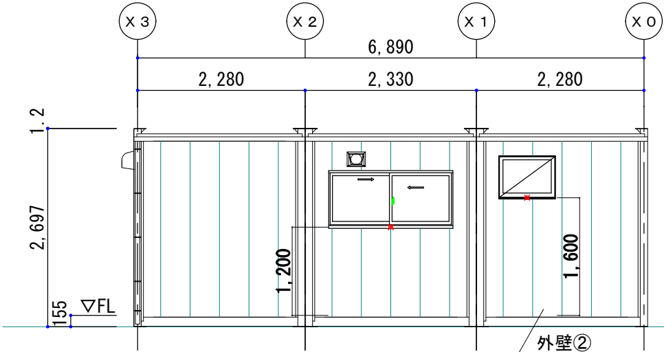
Y1通り 1/100
