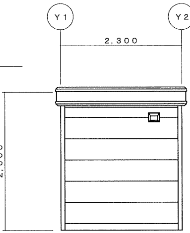
X2 立面図
