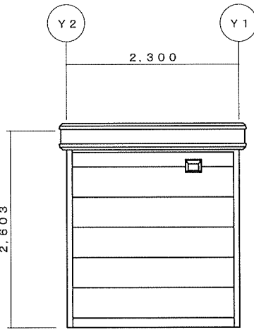
X1 立面図
