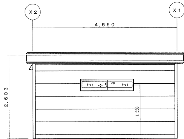
Y2 立面図
