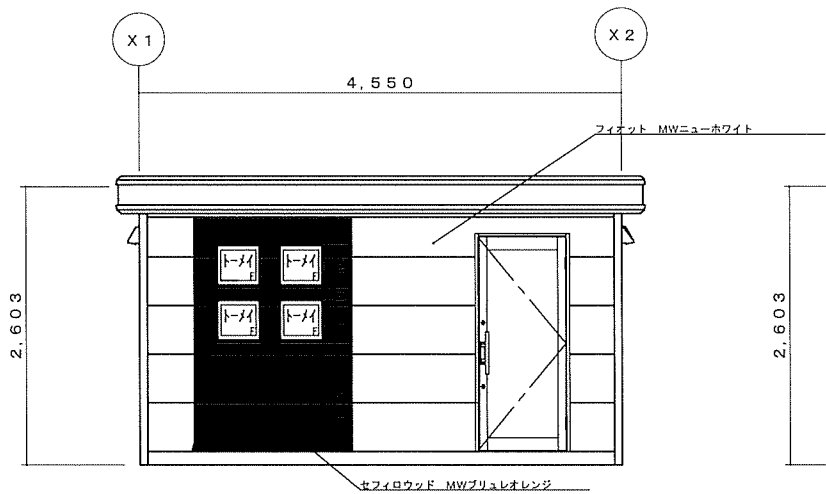
Y1 立面図
