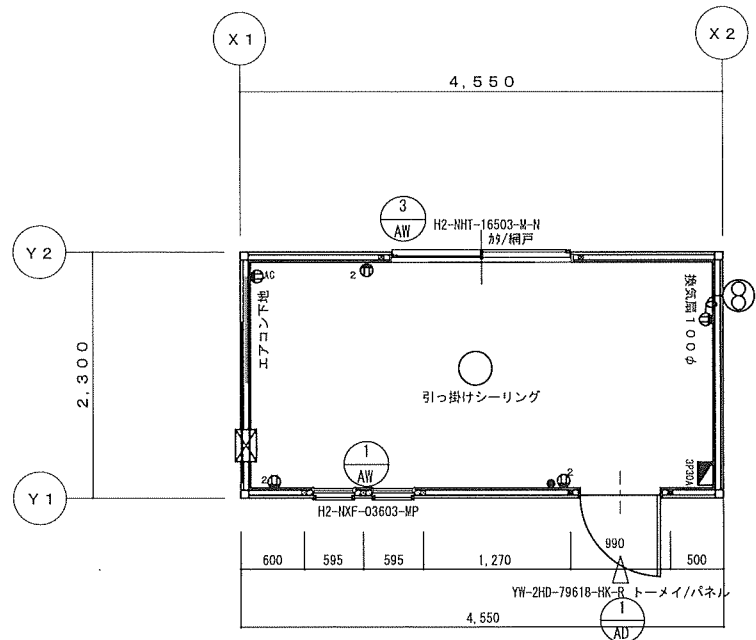
平面図
